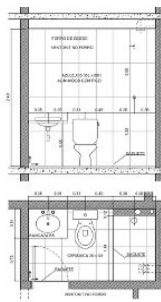
BANHOS PAV. TIPO UNIDADES 1
