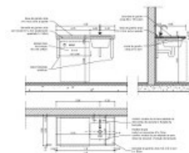
D04 - bancadas das cozinhas ESCALA 1:20
