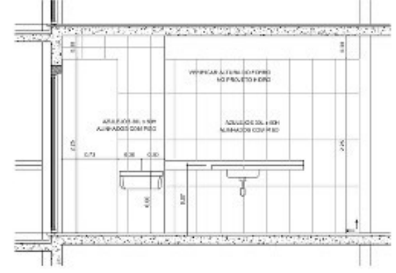
BANHOS PAV. TIPO UNIDADE 4 (2)
