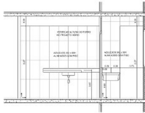
BANHOS PAV. TIPO UNIDADE 4 (1)
