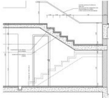
D17 - escada exterior térreo ESCALA 1:20
