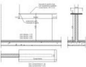
D01 D02 D03 - bancadas ESCALA 1:20
