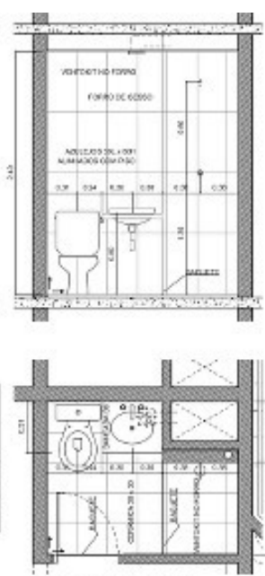
BANHOS PAV. TIPO UNIDADE 4 (2)
