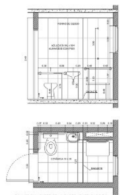
BANHOS PAV. SUPERIOR UNIDADES ADAPTADAS 2 E 3
