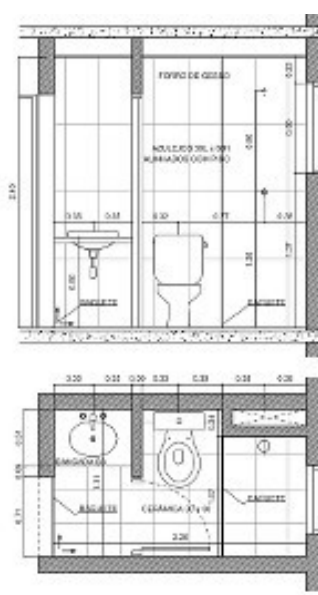
BANHOS PAV. TIPO UNIDADES 2 E 3
