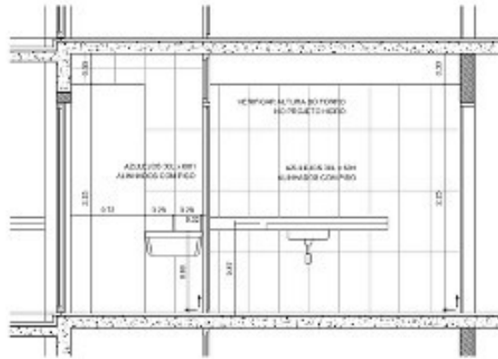
BANHOS PAV. TIPO UNIDADES 2 E 3
