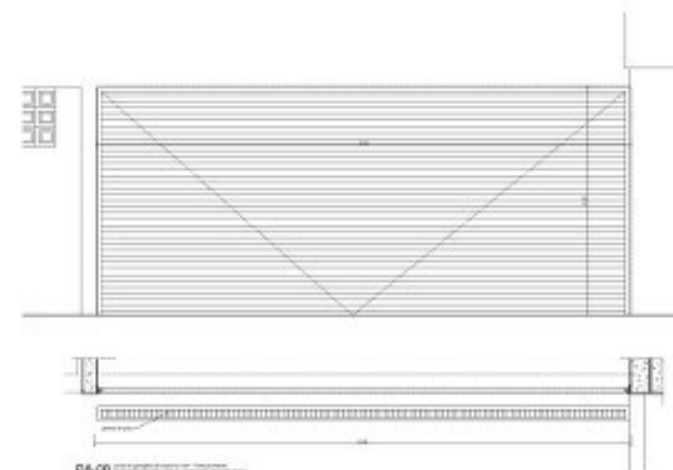
PA-08 ESCALA 1:20
